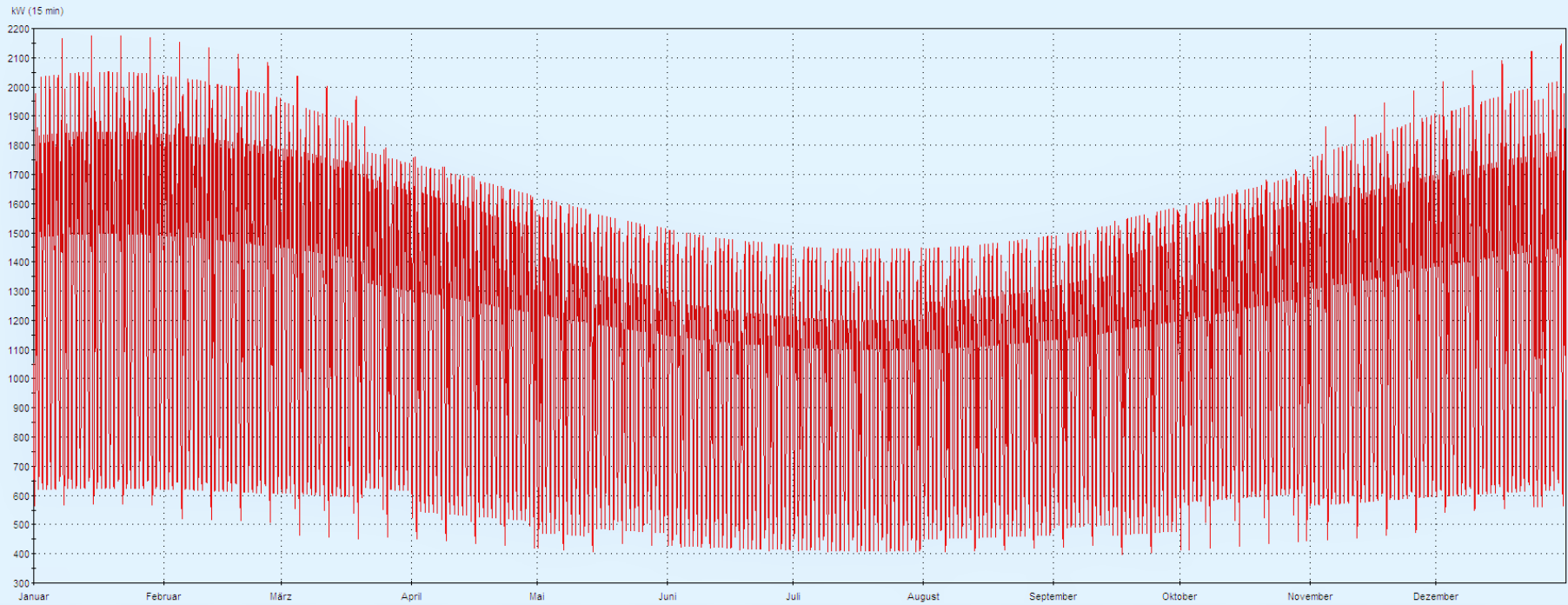
Summenlast Fahrplanprognose SLP-Kunden 2017
